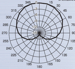
■ 参考 Reference (標準指向特性) (Standard Polar Pattern) Distance of 50cm, 1kHz
