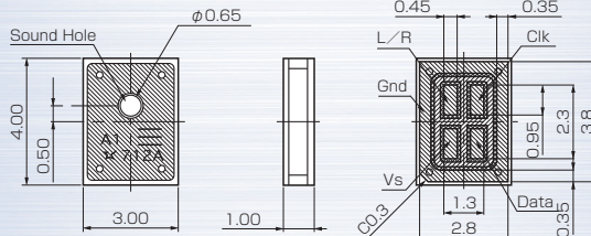
■ 外形寸法図 Dimensions
